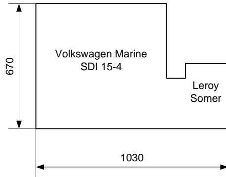
ZIJAAANZICHT
