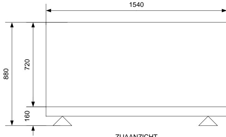
ZIJAAANZICHT
